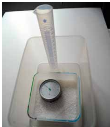
Abb. 8: Art sorb Granulat, Hygrometer und Messgefäß mit destilliertem Wasser (Foto: TLM)
